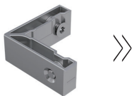
フレームの合番を合わせコーナー金物でジョイント
