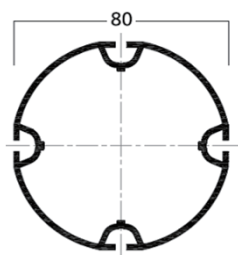
ROUND EXTRUSION - 80mm 丸形プロフィール 80mm
