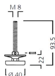
ADJUSTABLE FOOT アジャスター
