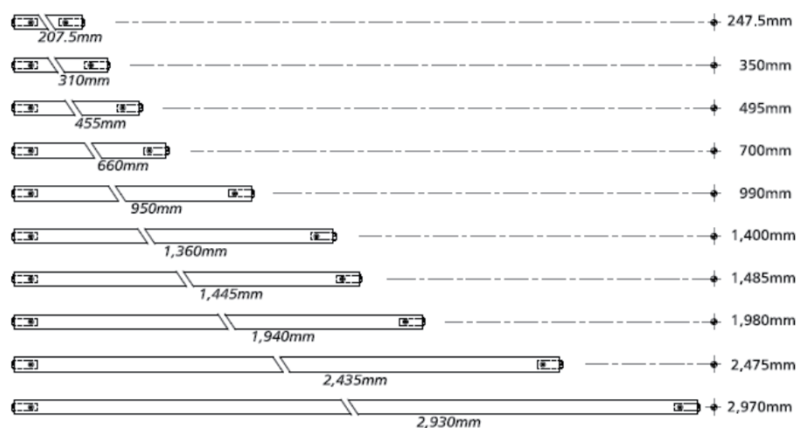
Beam extrusion 50mm ビーム 50mm
