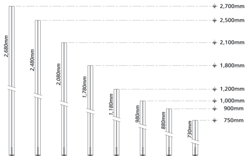
Upright - cut to size with Adjustable foot M1016 mounted アップライトポール・アジャスターM1016付
