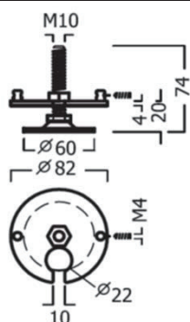
ADJUSTABLE FOOT アジャスター
