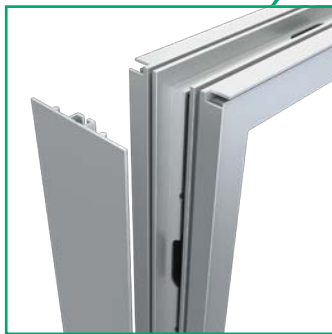
カバープロファイルの 取り付けが可能です
